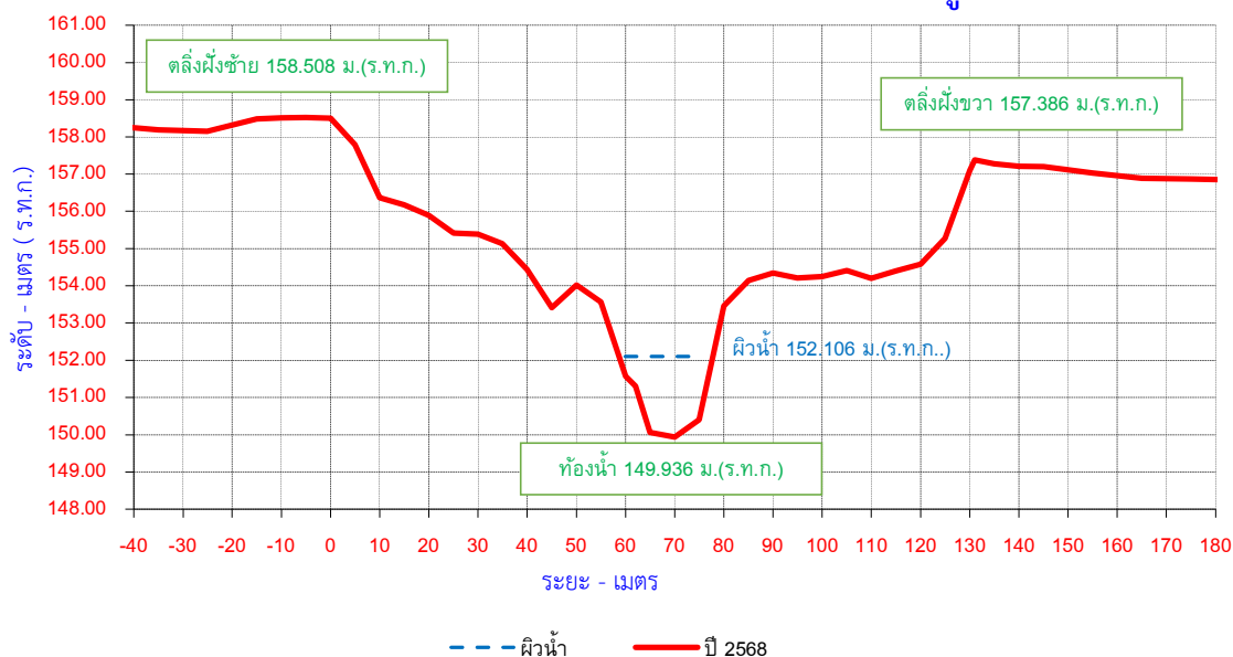
รูปตัดขวางลำน้ำ ปีน้ำ 2568 สถานี S.53 แม่น้ำป่าสัก อ.หล่มสัก จ.เพชรบูรณ์
